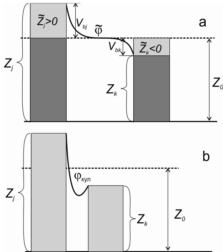
Рис.1. Схема возможного распределения потенциала между одноименно заряженными частицами: а – дальнейе притяжение частиц, б – ближнее кулоновское отталкивание.
