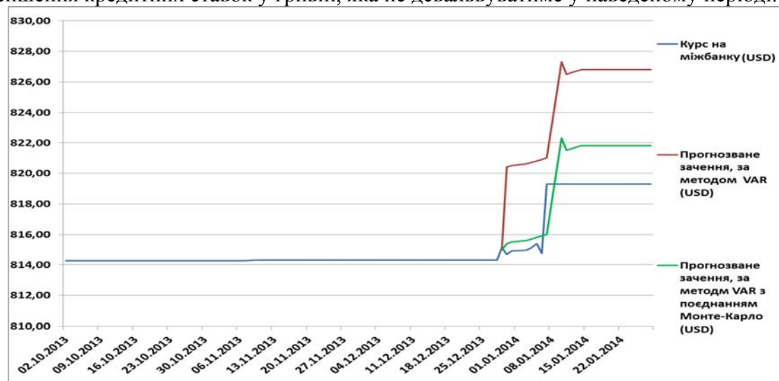
Рис. 2 Прогнозований курс долара до гривні за методикою VAR-аналізу на міжбанку
