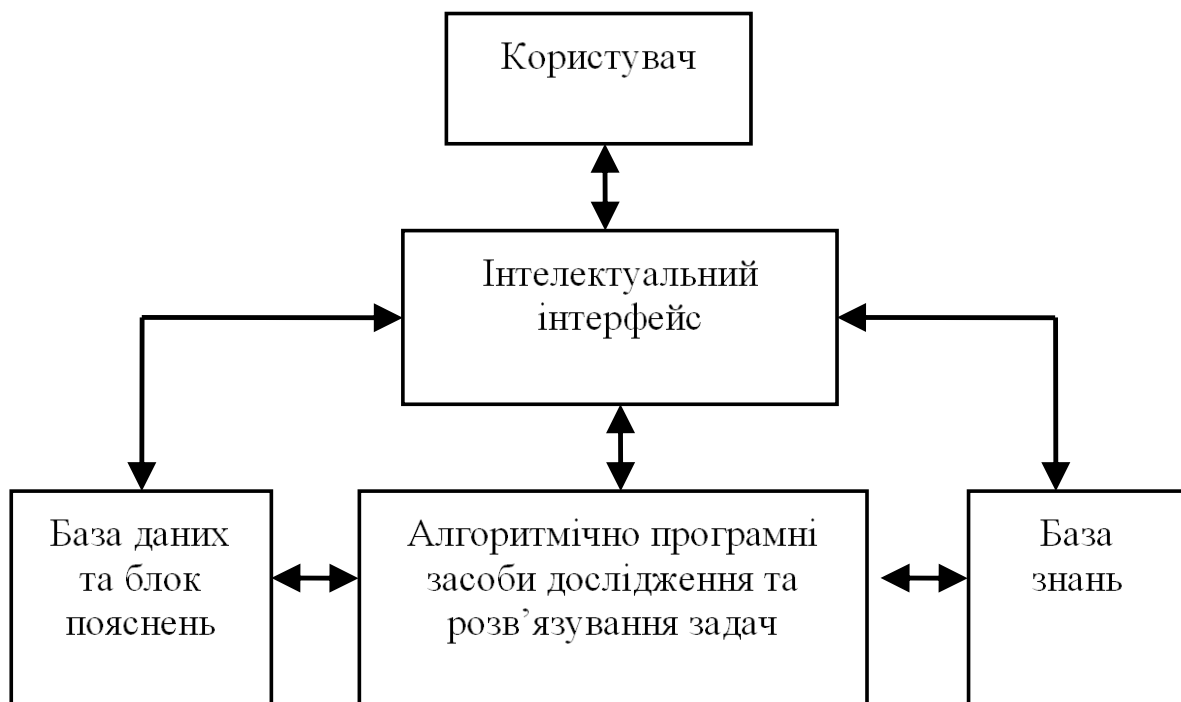
Рис. 1. Структура InparSolver
