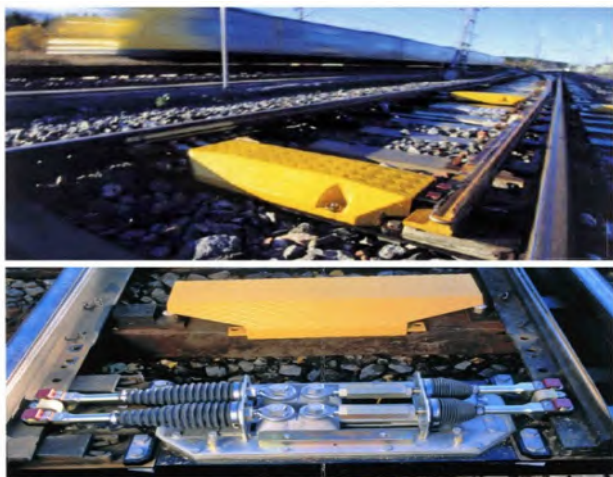
Рис.2. Система Hydrostar
