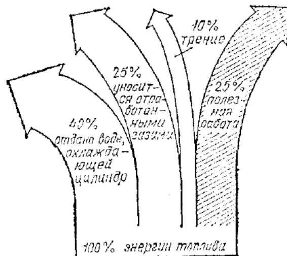
Рис. 1. Енергетичний баланс автомобільного двигуна
