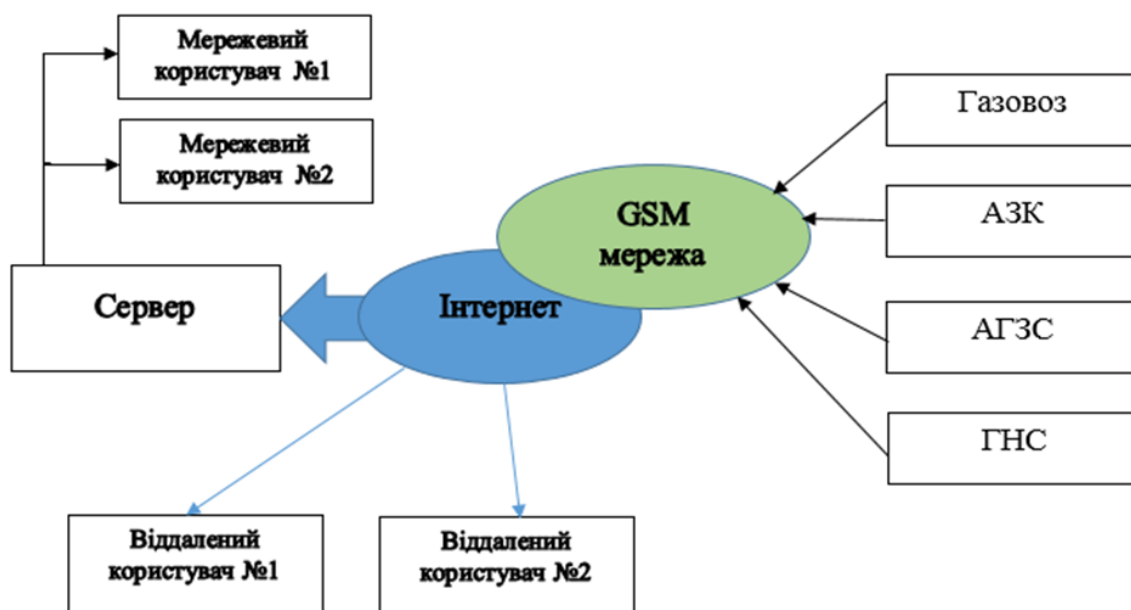
Рис. 1. Розподілена ІВС для обліку СВГ
