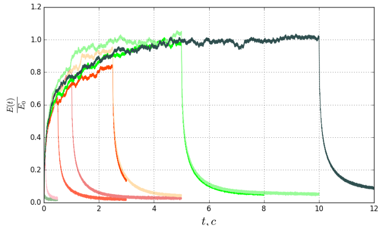
Рис. 3. Перехідні характеристики терморпарі за різної тривалості дії квазіступінчатого лазерного променя [8, 14 - 15]
