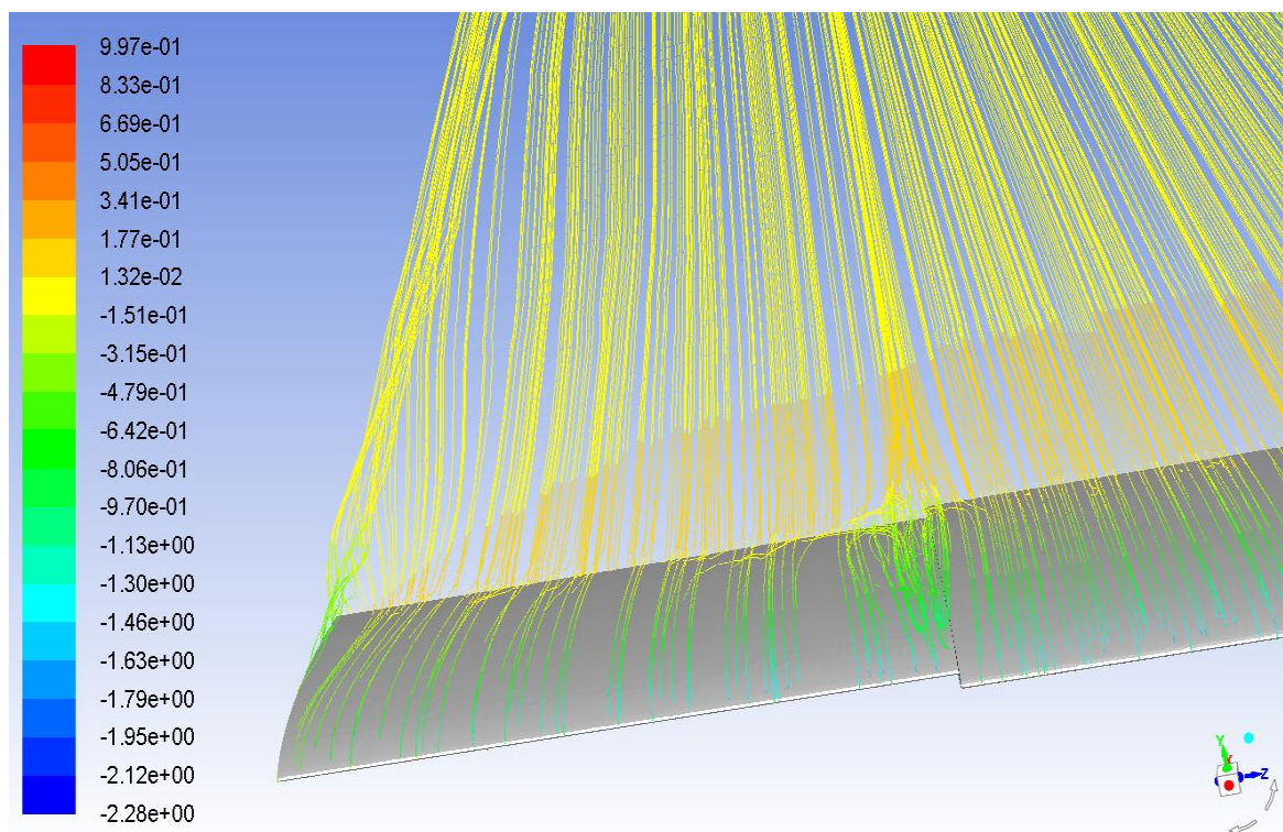
Рис. 9. 40% базового розмаху, кут атаки 8^\circ
