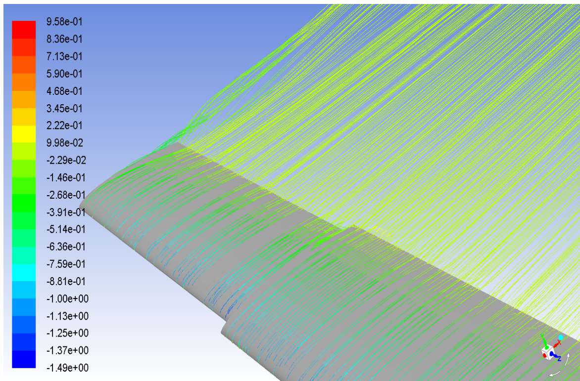
Рис. 8. 40% базового розмаху, кут атаки 6^\circ
