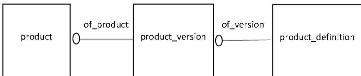
Рисунок 1 – Сутності продукту [7]
