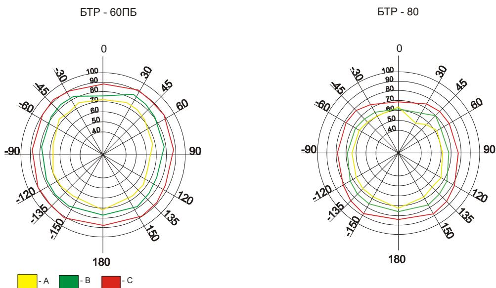
Рисунок 5 – Полярні діаграми
