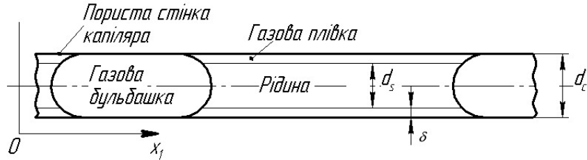
Рис. 1. Схема руху двухфазного середовища в снарядному режимі
