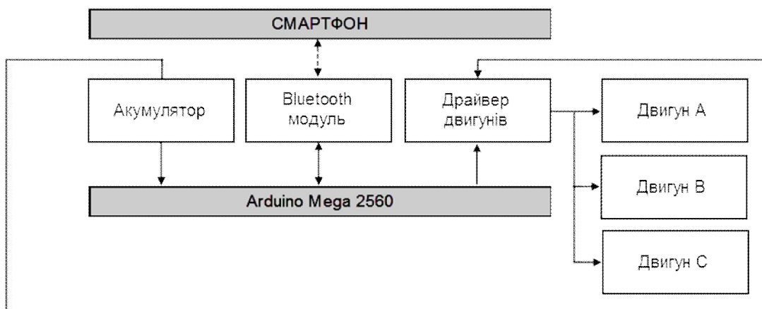
Рис. 4. Структура системи дистанційного управління роботом
