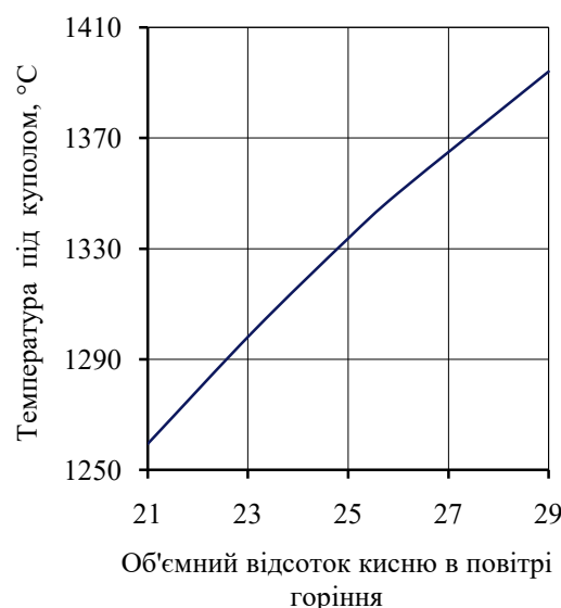
Рис. 2. Залежність температури під куполом від вмісту кисню в повітрі горіння
