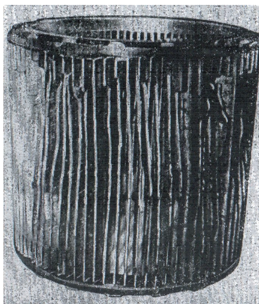
Рис. 2. Брак «беличьей клетки»
