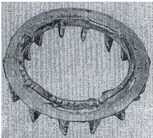
Рис. 3. Усадка от неполного заполнения кольца
