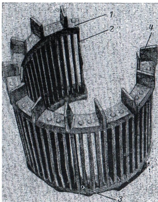
Рис. 1. «Беличья клетка». 1 – верхнее короткозамыкающее кольцо; 2 – стержень; 3 – нижнее короткозамыкающее кольцо; 4 – лопатка
