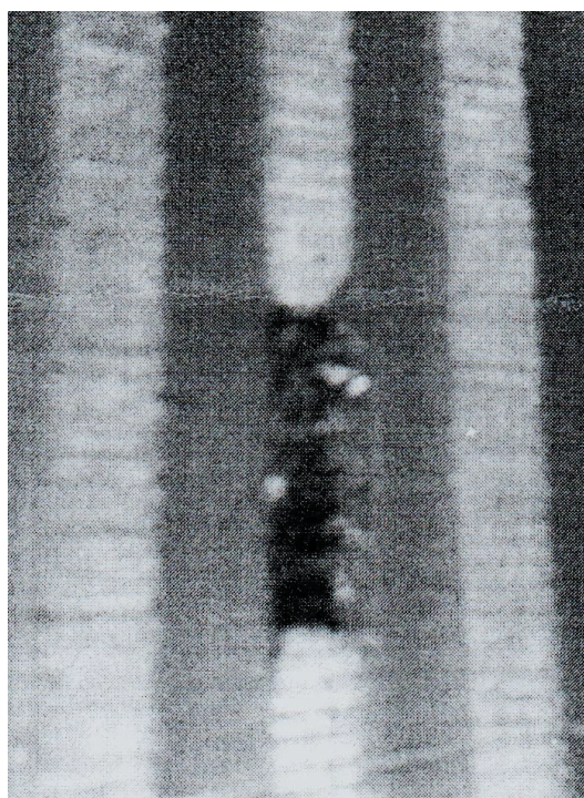
Рис. 5. Брак стержня «беличьей клетки»
