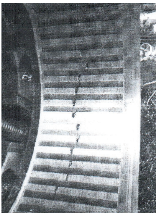
Рис. 4. Брак роторной обмотки
