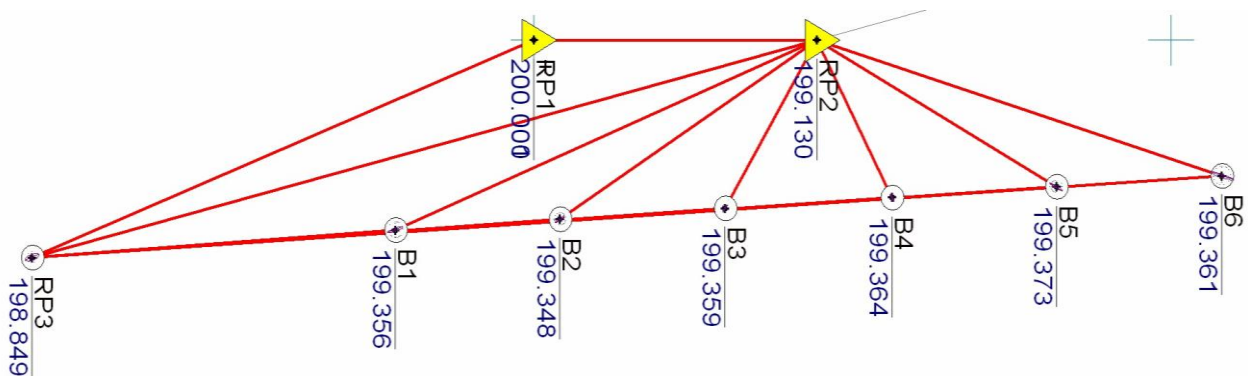
Рис. 3 Схема спостережень за осіданнями методом тригонометричного нівелювання.
