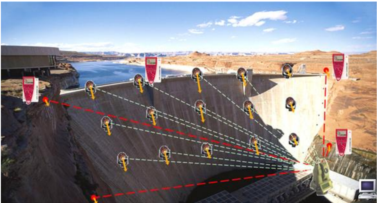
Рис. 10. Приклад встановлення системи автоматизованого геодезичного моніторингу
