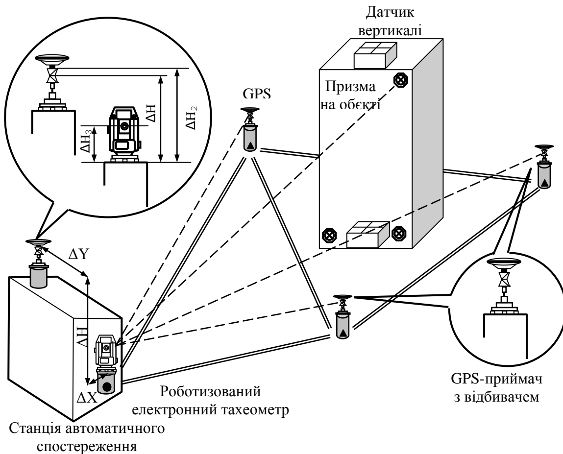
Рис. 9 Структурна схема системи автоматизованого геодезичного моніторингу
