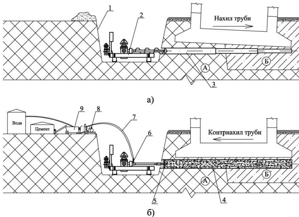
Рис. 1 – Технологічна схема відновлення деформованої нахиленої димової труби: а) буріння лідерної горизонтальної ступінчатої свердловини при вирівнюванні труби; б) утворення горизонтального армуючого ґрунтоцементного елемента при підсиленні основи; А – мергелястий ґрунт; Б - насипний ґрунт; 1 – котлован; 2 – станок горизонтального буріння; 3 – горизонтальна свердловина; 4 - горизонтальний ґрунтоцементний армоелемент; 5 - розбурювач; 6 – вертлюг; 7 – рукав; 8 – розчинонасос; 9 – розчиномішалка.
