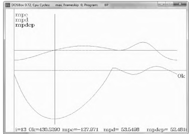
Рис.12.Графіки приведених моментів сил опору (зелена крива),моменту двигуна (червона крива) и середнього моменту рушійних сил (бузкова крива)
