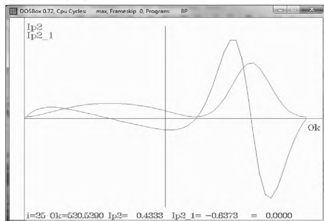
Рис.8. Графіки приведенного моменту інерції ланок механізму (зелена крива у кг·м 2 ) і першої похідної за УК(червона крива)
