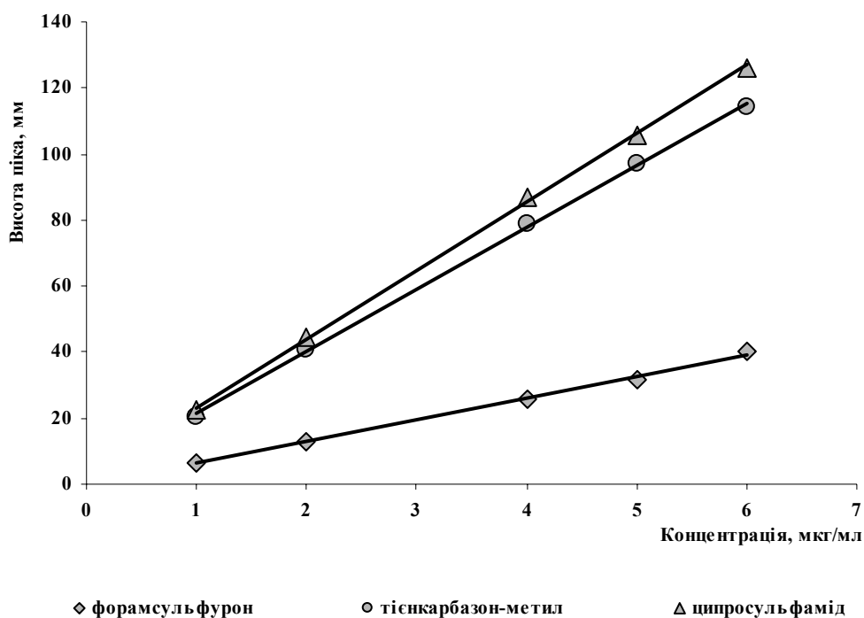
Рис. 2. Градувальні залежності висоти хроматографічного піка форамсульфурону, тієнкарбазон-метилу та ципросульфаміду (мм) від концентрації у градуювальному розчині (мкг/мл)
