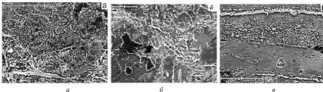
Рис. 2. Мікроструктура компактів, що були спечені при різних початкових тисках: a - P_1 = 0,5 МПа, b - P_2 = 3 МПа, v - P_3 = 9,5 МПа
