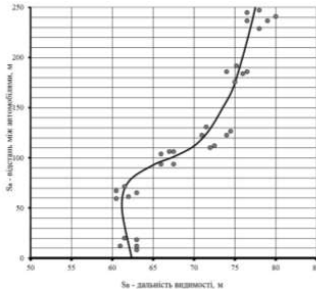
Рис. 4. Залежність дальності видимості від відстані між автомобілями
