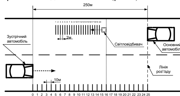
Рис. 3. Розташування транспортних засобів на початку експерименту
