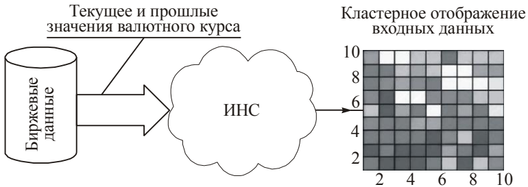
Рис. 8. Решение задачи валютного дилера как задачи кластеризации
