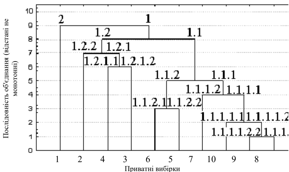
Рис. 5. Дендрограма результатів кластеризації зваженим центроїдним медіанним методом ділянок по вмісту Ge. Умовні позначення: 1, 2, 1.1, 1.2, 1.1.1, 1.1.2, 1.1.1.1, 1.1.1.2, 1.2.1, 1.2.2, 1.2.1.1, 1.1.2.1, 1.1.2.2, 1.1.1.1.1, 1.1.1.1.2, 1.1.1.1.2.1, 1.1.1.1.2.2 – кластери
