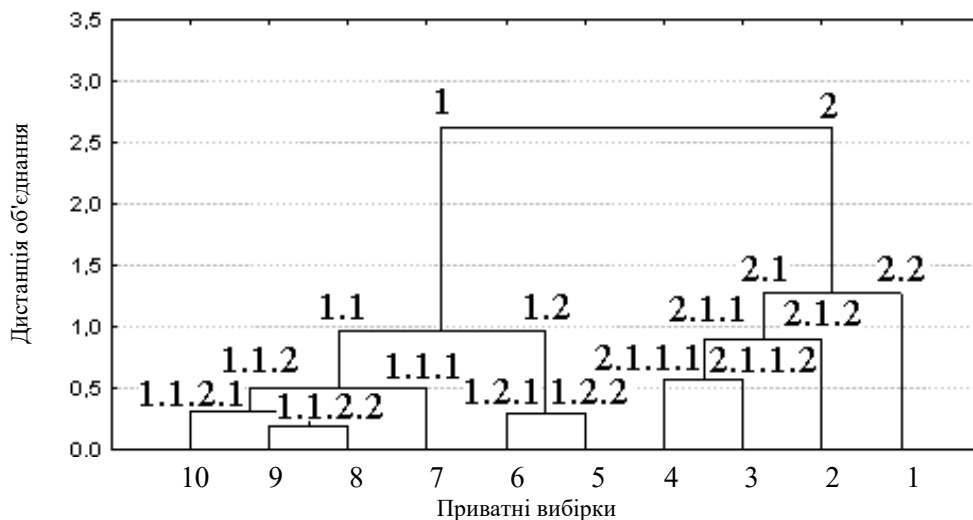
Рис. 2. Дендрограма результатів кластеризації методом повного зв'язку ділянок по вмісту Ge. Умовні позначення: 1, 2, 1.1, 1.2, 1.1.1, 1.1.2, 1.1.2.1, 1.1.2.2, 1.2.1, 1.2.2, 2.1, 2.2, 2.1.1, 2.1.2, 2.1.1.1, 2.1.1.2 – кластери
