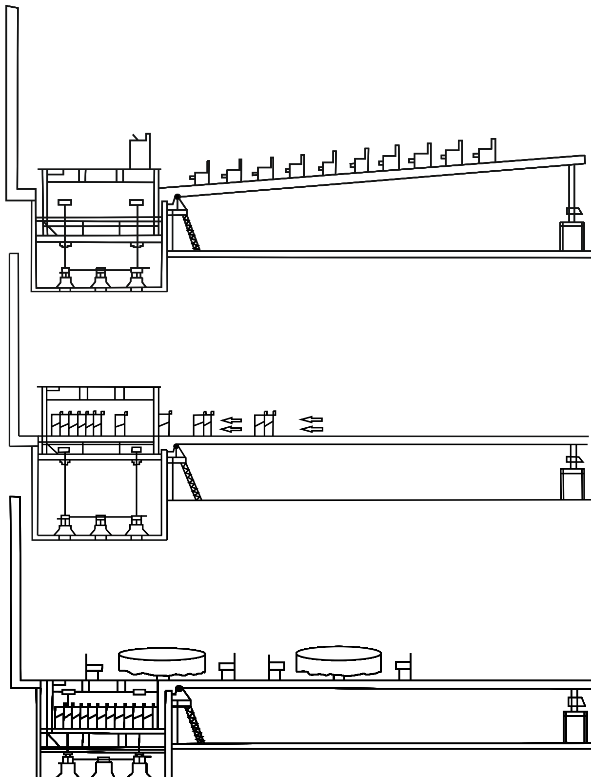
Рис.1. Автоматична пересувна система крісел
