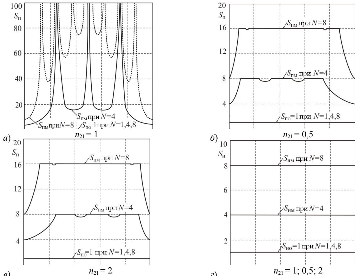
Рисунок 9 – Зависимости коэффициентов сглаживания структуры по току на входе S_{оп} , S_{мп} и выходе S_{он} , S_{нп} соответственно ОИП и МИП
