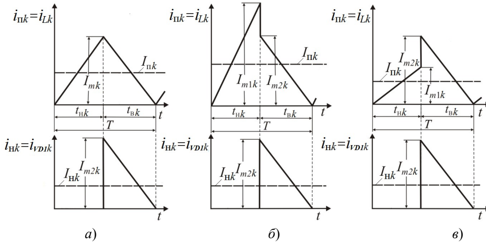
Рисунок 3 – Временные диаграммы токов потребления i_{пк}(t) и нагрузки i_{нк}(t) k -го ( k = 1 ) СК в граничном режиме функционирования при n_{21} = 1 (а); n_{21} > 1 (б); n_{21} < 1 (в) при U_n = \text{const}
