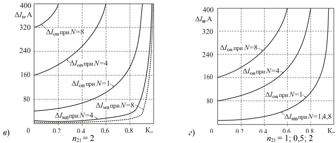
Рисунок 6 – Зависимости размахов пульсаций во входных (а, б, в) и выходных (г) цепях ОИП и МИП при P_{нк} = 200 Вт и P_n = P_{нк}N
