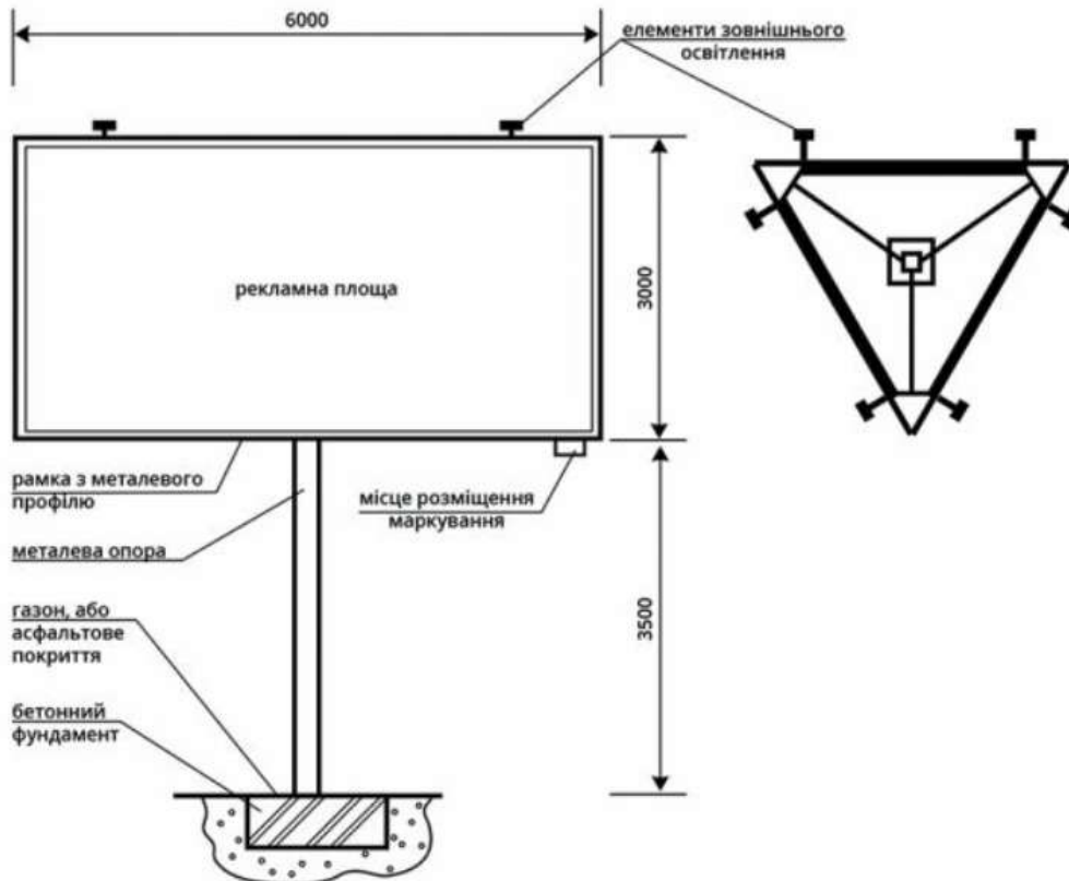
Рисунок 4 – Білборд типу 3
