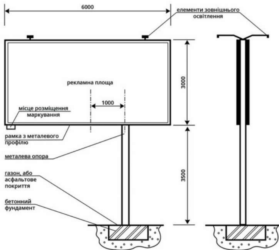
Рисунок 2 – Білборд типу 1
