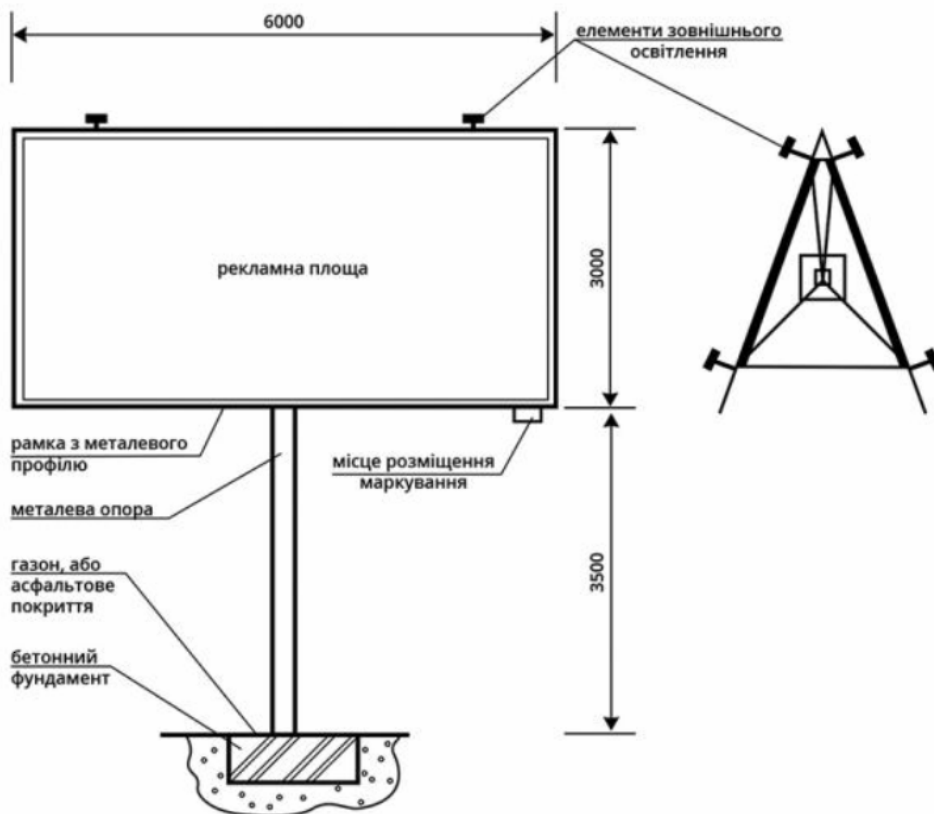
Рисунок 3 – Білборд типу 2
