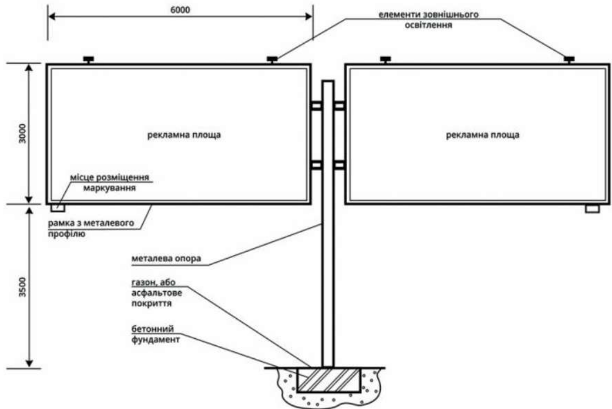
Рисунок 5 – Білборд типу 4
