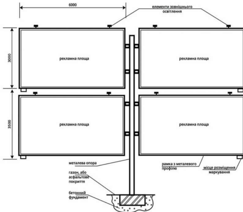
Рисунок 6 – Білборд типу 5
