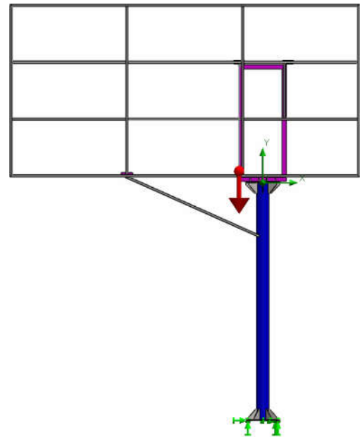
Рисунок 10 – Граничні умови
