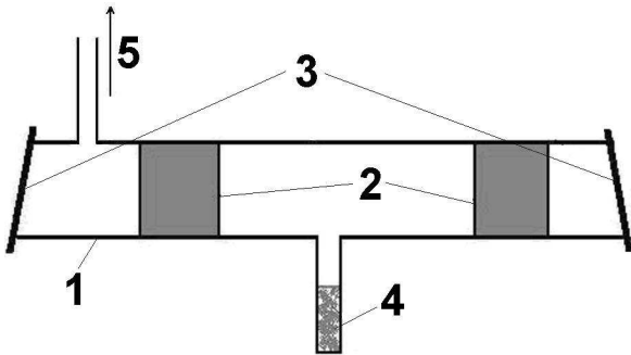
Рис. 1. Конструкція електророзрядної лампи на парах води і перекису водню, де 1 – кварцова трубка, 2 - танталові електроди, 3 – вихідні вікна, 4 – суміш води і перекису водню, 5 - відкачка ГРТ.
