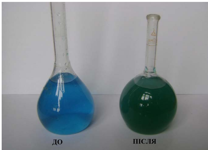
Рис.2. Вигляд розчину мідного купоросу до і після обробки поверхні електроліту сильнострумиви наносекундним розрядом.
