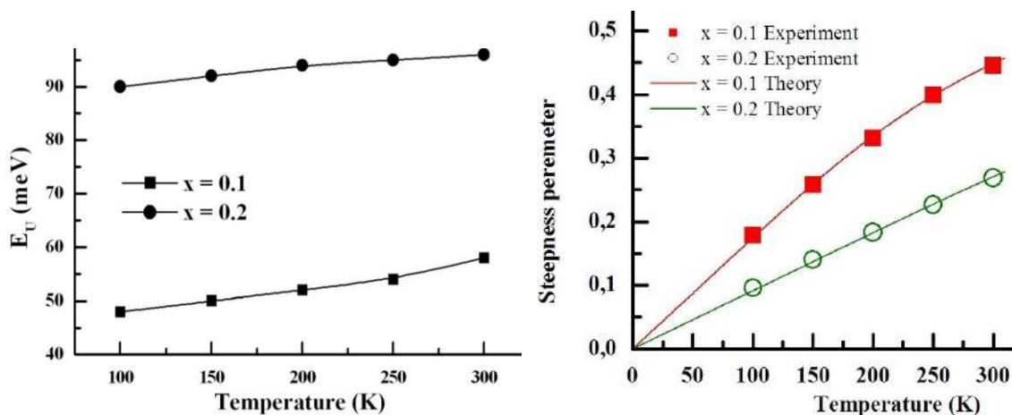
Рис. 3. Залежність енергії Урбаха E_U (а) та параметра крутизни \sigma(T) (б) монокристалів Tl_{1-x}In_xSi_xSe_2 від температури
