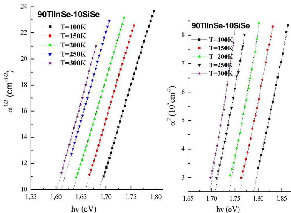
Рис. 2. Спектральна залежність (\alpha hv)^{1/2} (а) і (\alpha hv)^2 (б) для \text{Tl}_{1-x}\text{In}_{1-x}\text{Si}_x\text{Se}_2 ( x=0,1 ) монокристалів за різних температур
