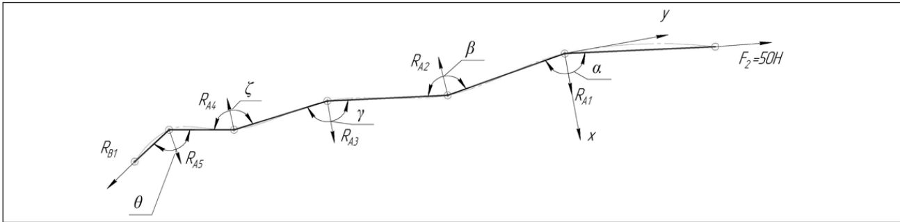
Рис. 3. Схема міжсегментарних кутів та реакцій від сили натягу ізолюваного сухожилка глибокого згинача пальця в системі координат X0Y
