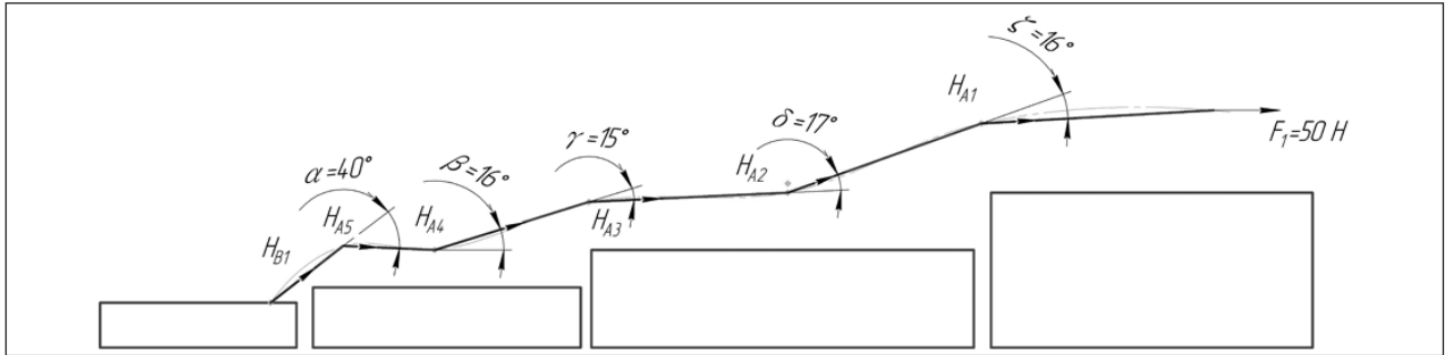
Рис. 4. Розрахункова схема
