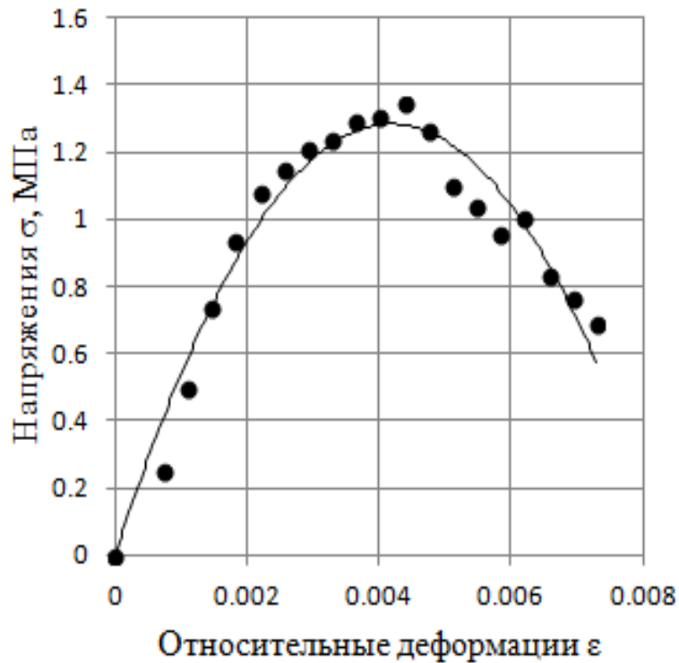
Рис. 2. Диаграмма физического состояния грунтоцемента
