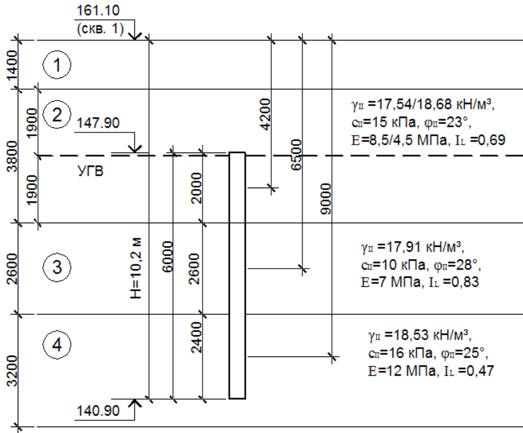
Рис. 1. Расчетная схема свай
