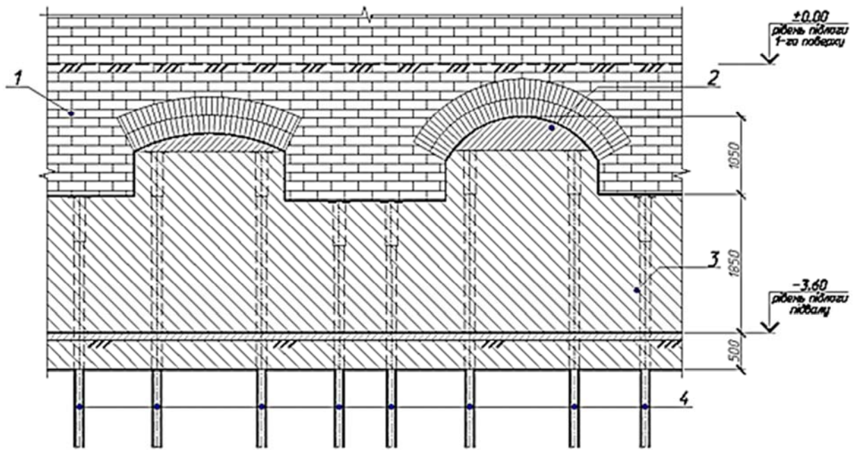
Рис. 3. Фрагмент ділянки підсилення з-під підшови фундаментів: 1 – існуючий фундамент з розвантажувальними арками; 2 - розподільча балка; 3 – залізобетонне нарощування стіни підвалу; 4 – вдавлювані палі
