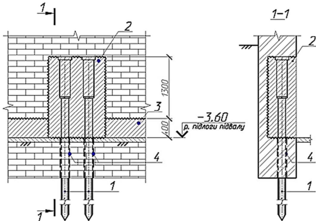
Рис. 2. Фрагмент ділянки підсилення з ніш в цегляній кладці: 1 – вдавлювані палі; 2 – ніша, омонолічена з оголовками палей; 3 – залізобетонний пояс; 4 – отвори в кладці фундаменту
