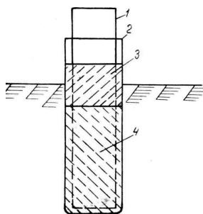
Рис. 1.3. Схема диференційованого просочування стовпа у підставній ванні: 1 – стовп; 2 – поліетиленова плівка; 3 – розчин захисного засобу; 4 – водний розчин
