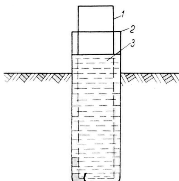
Рис.1.2. Схема просочування стовпа в підставній ванні: 1 – стовп; 2 – поліетиленовий мішок; 3 – просочувальний розчин
