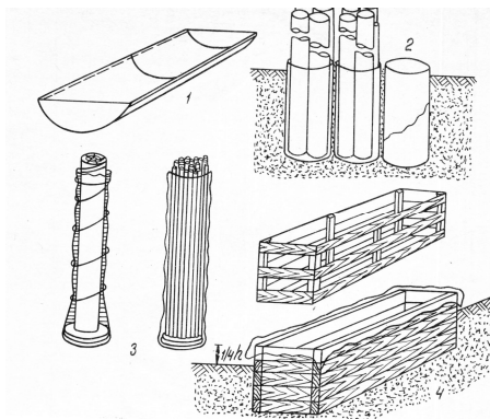
Рис.1.1. Тимчасові ванни для просочення невеликих партій деревини: 1 – зварна горизонтальна ванна із сталевих бочок; 2 – просочення круглих стійок в бочках, вкопаних в ґрунт; 3 – просочення стійок в поліетиленових мішках; 4 – дерев'яна ванна, що вистелена поліетиленовою плівкою
