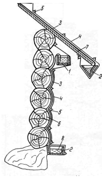
Рис.1.5. Схема панельного просочування колодчастої стінки і гонтової покрівлі:
