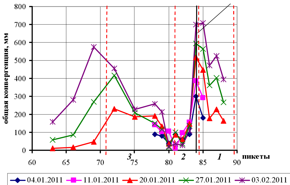
Рис. 4. Общая вертикальная конвергенция ЮМОШ № 3 при отходе лавы от разрезной печи
