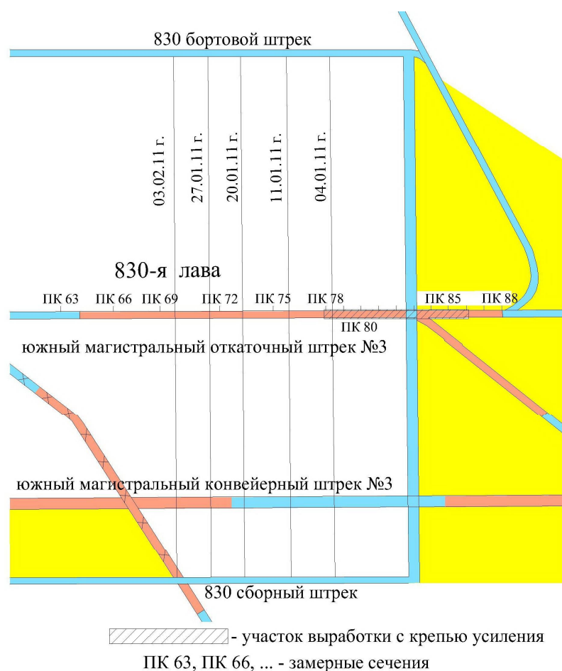
Рис. 3. Выкопировка из плана горных работ по пл. с шахта «Западно-Донбасская»
