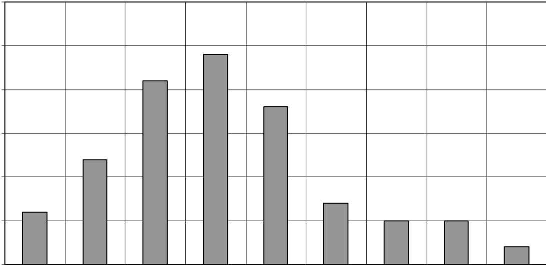
Рис. 1. Распределение отклонений фактических размеров целиков от проектных
