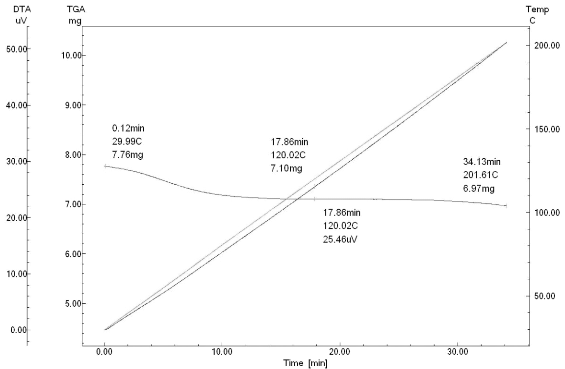
Рис. 3. Дериватограма карбополу.
