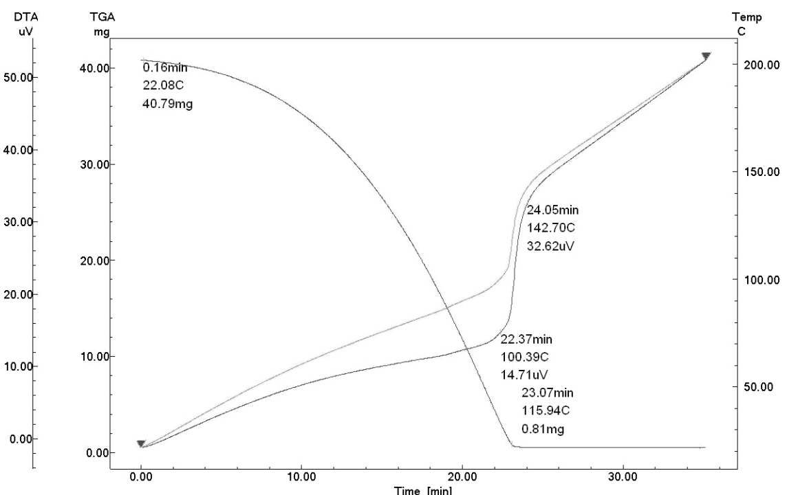
Рис. 4. Дериватограма гідрофільної гелевої основи на основі карбополу.
