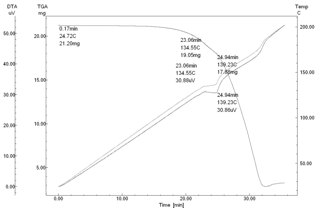
Рис. 2. Дериватограма консерванту – кислоти сорбінової.
