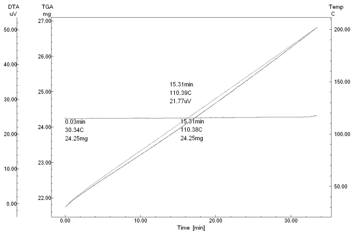
Рис. 1. Дериватограма активного фармацевтичного інгредієнта – таурину.
