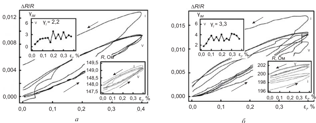
Рис. 3. Залежність \Delta R/R , R та \gamma_I від \epsilon_p для плівки Co(20)/Cu(30)/PI без (а) та при дії магнітного поля (б)
