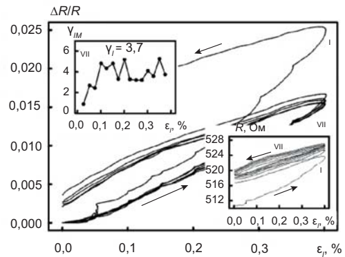
Рис. 2. Залежність \Delta R/R , R та \gamma_{II} від \epsilon_r для плівки Co(36)/П без (а) та при дії магнітного поля (б)
