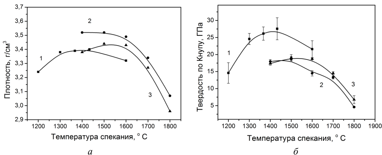
Рис. 1. Зависимость плотности (а) и твердости по Кнупу (б) от температуры спекания композитов различного состава: 1 – Q–50 % BN сф (нано); 2 – Q–30 % BN сф (субмикро); 3 – Q–50 % BN сф (субмикро)
