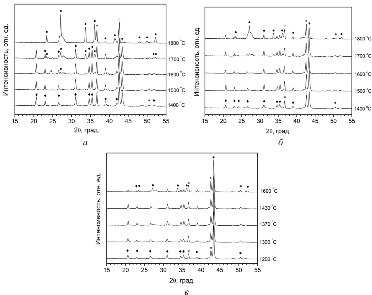
Рис. 3. Дифрактограммы композитов Q с добавкой 30% (а), 50 % (б) BN_{cf} (субмикро), и 50% BN_{cf} (нано) (в), спеченных при различных температурах. ♦ – \alpha-Si_3N_4 ; ● – \beta-Si_3N_4 ; ○ – TiN; * – BN_{cf}
