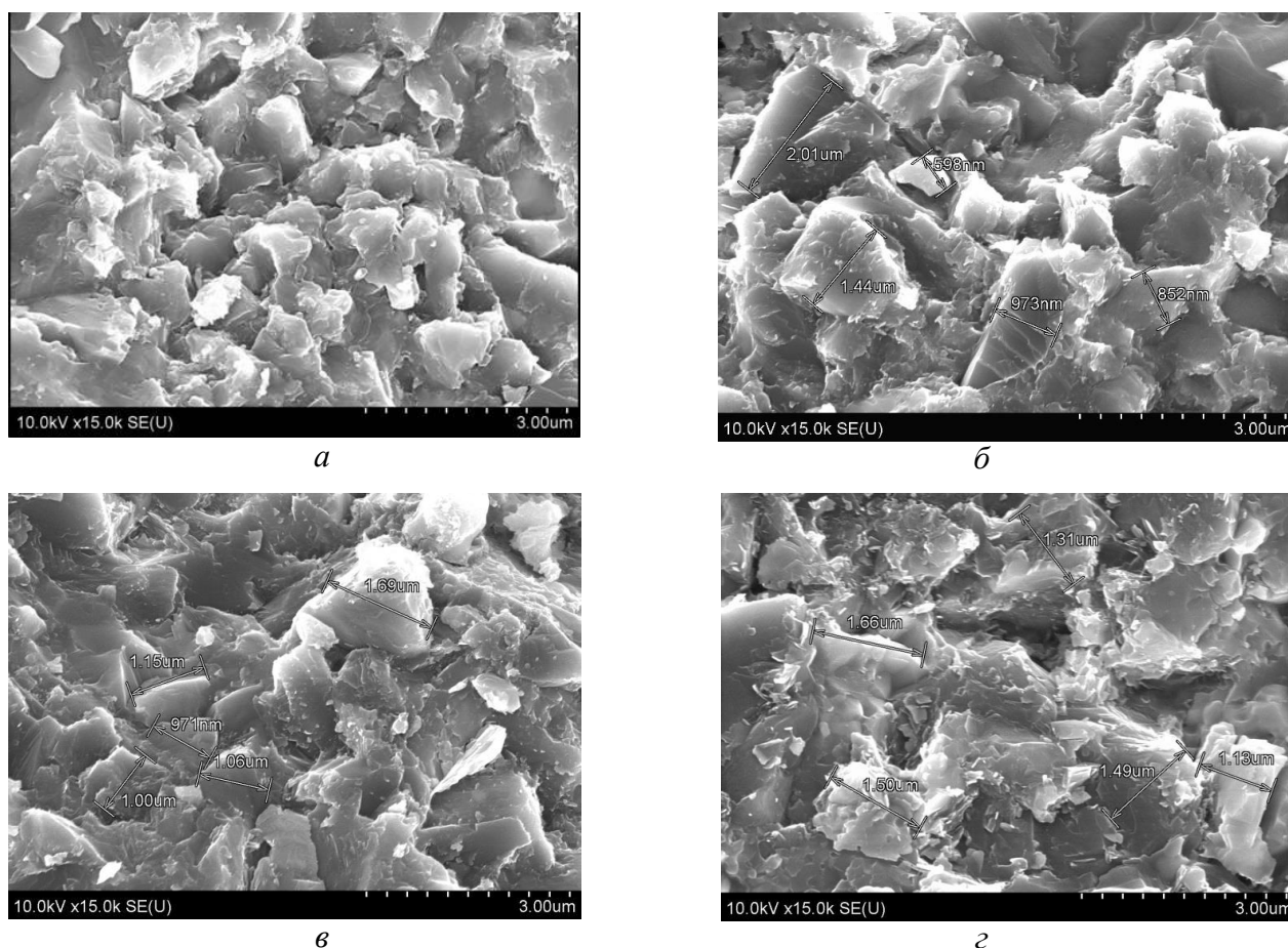
Рис. 4. Микрофрактограммы изломов образцов композита с добавкой 50 % \text{BN}_{\text{сф}} (нано), спеченных при различных температурах, °С: а – 1300; б – 1370; в – 1430; з – 1600.
