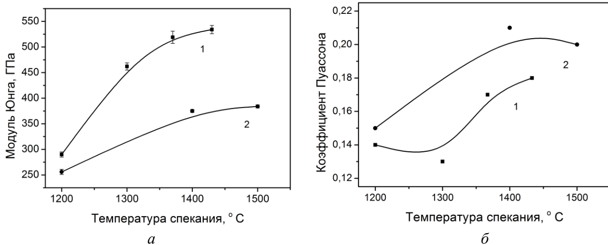
Рис. 2. Зависимости модуля Юнга (а) и коэффициента Пуассона (б) от температуры спекания композитов различного состава: 1 – Q–50 % \text{BN}_{\text{сф}} (нано); 2 – Q–30 % \text{BN}_{\text{сф}} (субмикро)
