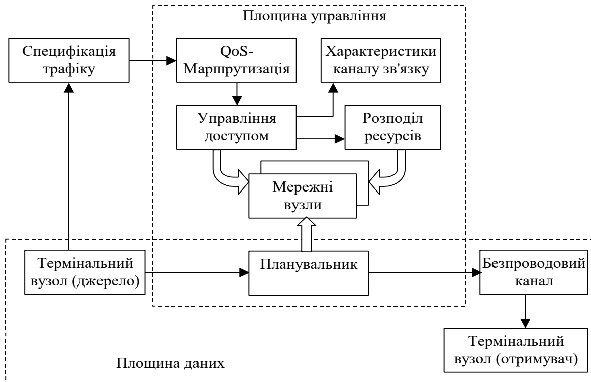
Рис. 1. Мережна архітектура для резервування QoS
