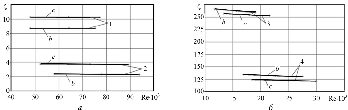
Рис. 2. Зависимость коэффициента местного сопротивления \zeta от числа Рейнольдса Re для диафрагм, установленных со стороны всасывания (b) и с напорной стороны (c) вентилятора при k = 0,38 (1), k = 0,65 (2), характерных для области малых (a), и k = 0,11 (3), k = 0,15 (4), характерных для области больших (б) сопротивлений
