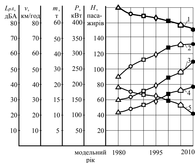
Рис. 1. Діаграма зміни у часі параметрів технічного рівня тролейбусів: 1 — нормативний рівень шуму L_{pA} ; 2 — максимальна швидкість v ; 3 — пасажиромісткість H ; 4 — потужність двигуна P ; 5 — маса t спорядженого тролейбуса; позначки відповідають моделям: \Delta — ЗиУ-682Б; \circ — ЗиУ-9; \square — ЮМЗ-Т2; \diamond — ЛиАЗ ТР 5280; \blacksquare — МАЗ-СВАРЗ; \triangle — Тролза Megapolis; \bullet — Богдан Т701.15
