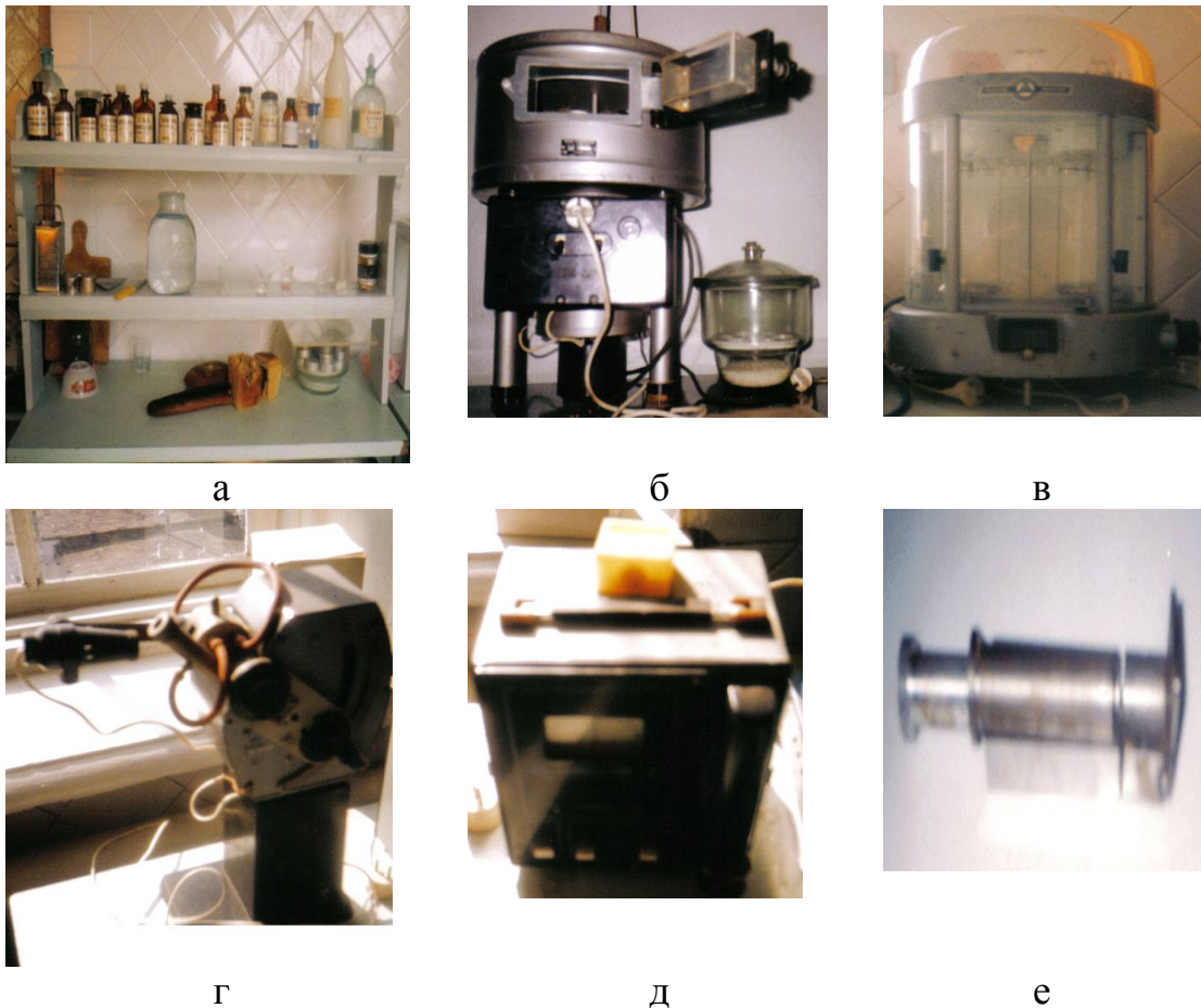
Рис. 1. Прилади для контролю процесів тістоприготування: а – прилади для виміру титрованої кислотності; б – ВПШП-4 (сушильна електрошафа з терморегулятором Чижової); в – аналітичні ваги ВЛА-200г-М з точністю до 0,001 кг.; г – позиційний профілактометр УРЛ-Модуль1; д – прилад ІДК-1; е – прилад Журавльова.
