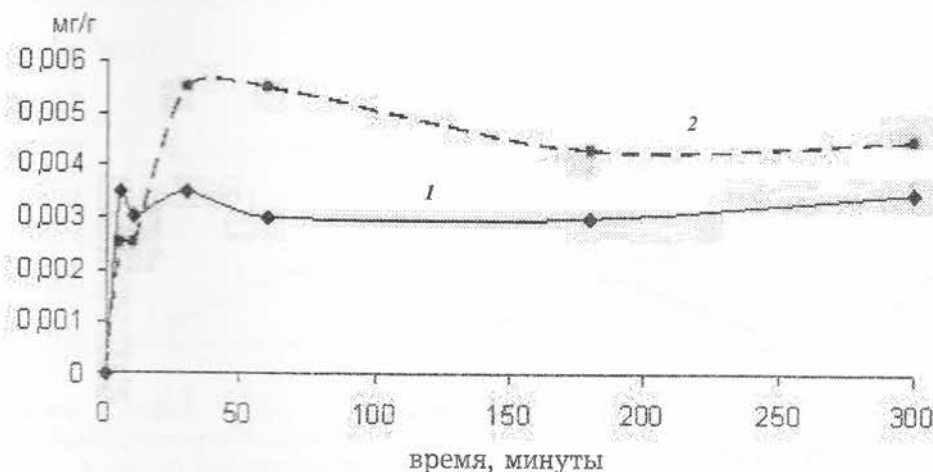
Рис. 2. Сорбция каолинитом лития из растворов Li 2 SO 4 . Концентрация Li, мг/л: 1 - Li - 5, 2 - Li - 10
