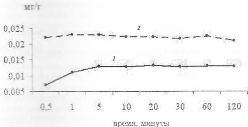
Рис. 6. Десорбция природного лития из почвы. Экстрагенты: 1 — 0,05 н HCl; 2 — 1 н HCl
