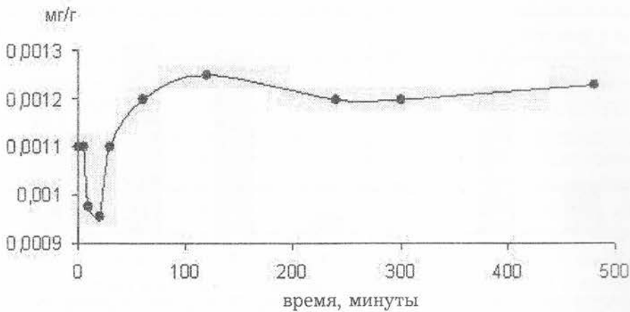
Рис. 3. Десорбция природного лития из монтмориллонита 0,01 н раствором HCl
