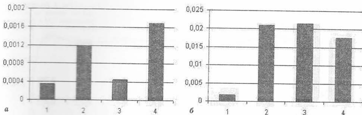
Рис. 1. Десорбция Li из природных глинистых минералов. 1 - каолинит, 2 - монтмориллонит, 3 - сапонит, 4 - иллит. Экстрагенты: а - H 2 O, б - 1 н HCl
