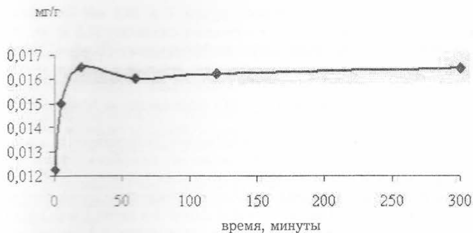
Рис. 5. Десорбция лития из сапонита 0,05 н раствором HCl
