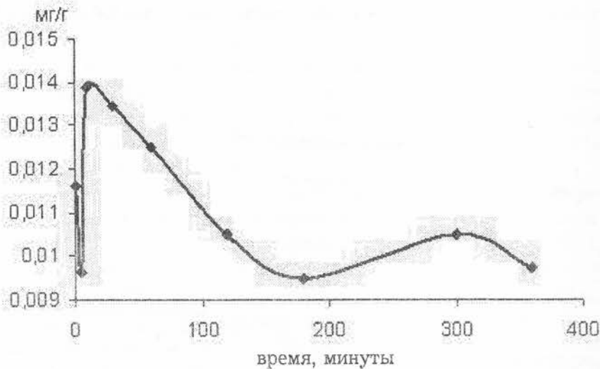
Рис. 4. Сорбция лития сапонитом из раствора Li_2SO_4 с концентрацией Li 5 мг/л
