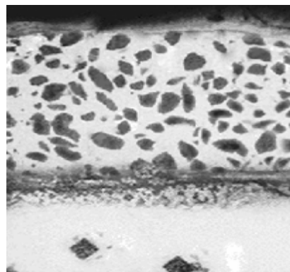
Рис. 3, б – Мікроструктура КЕП після дифузійного хромування \times 300
