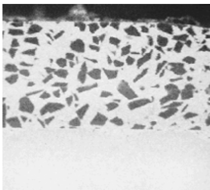
Рис. 3, а – Мікроструктура КЕП Ni-TiC з наповнювачем TiC \times 300
