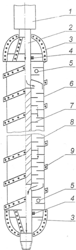
Рис. 4. Випрямляч стовбура свердловини
