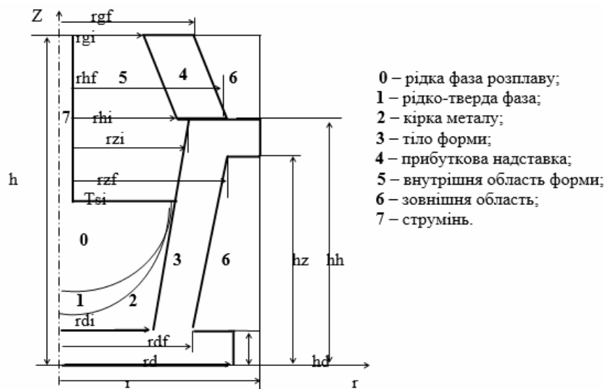
Рисунок 2 — Розрахункова область
