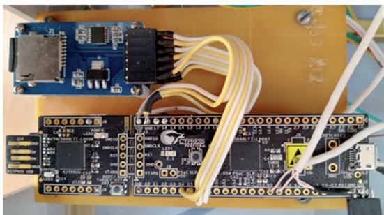
Формувач модульованих сигналів PSoc 5 LP
