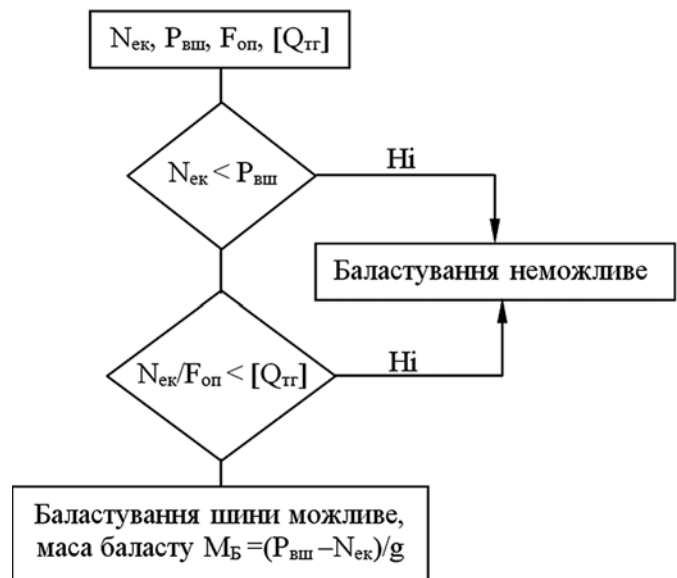
Рис. 1 – Блок-схема алгоритму визначення можливості баластування рушія колісного енергетичного засобу
