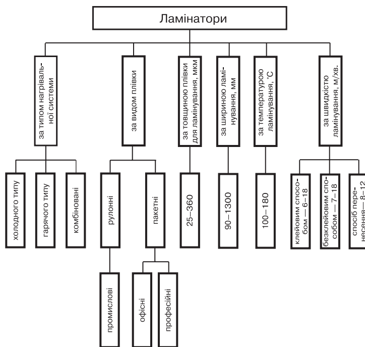
Рис. 2. Класифікація ламінаторів
