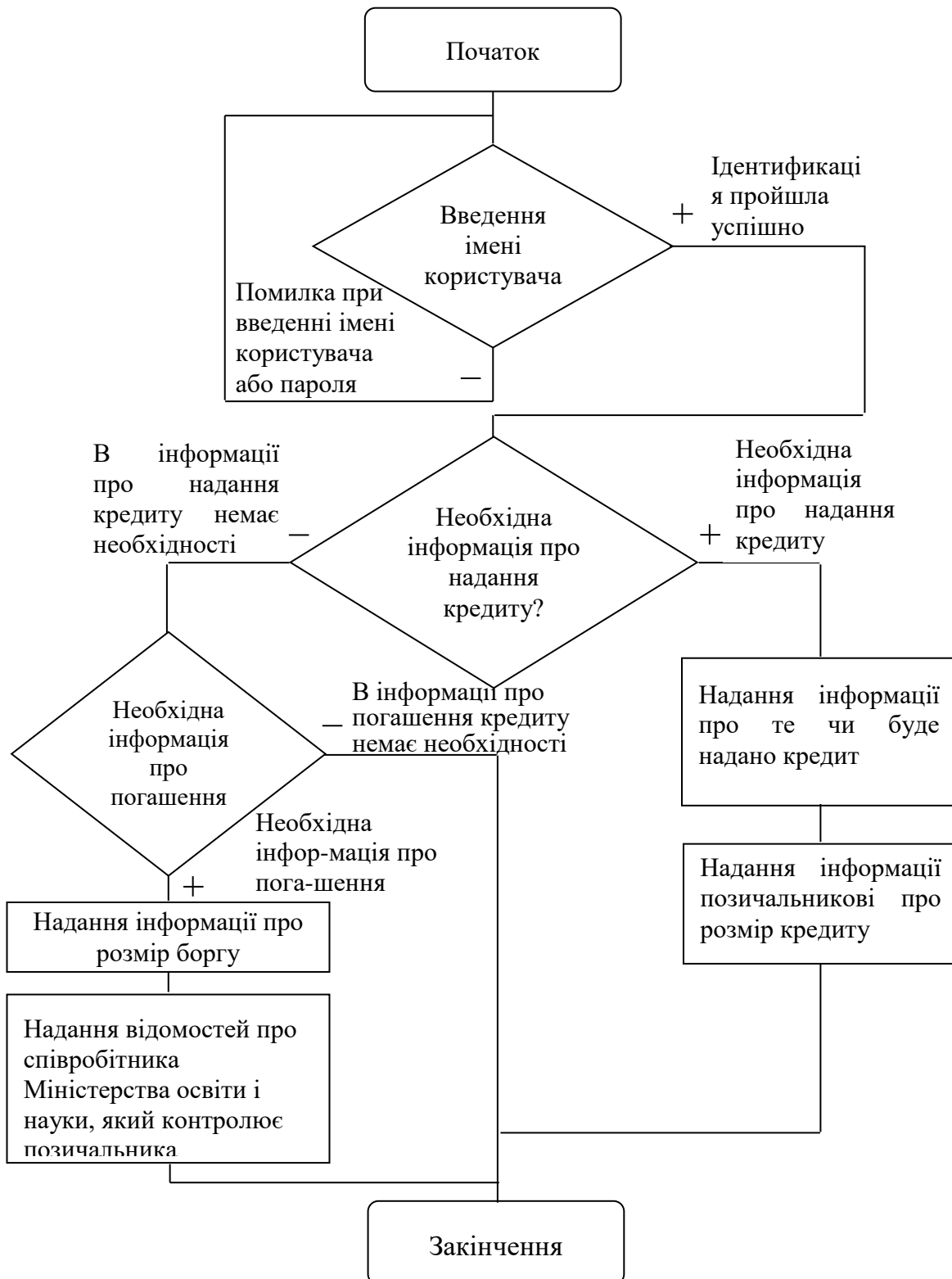
Рисунок 1 – Алгоритм взаємодії позичальника з багаторівневою інформаційною системою державного кредитування освітніх послуг через Internet-портал
