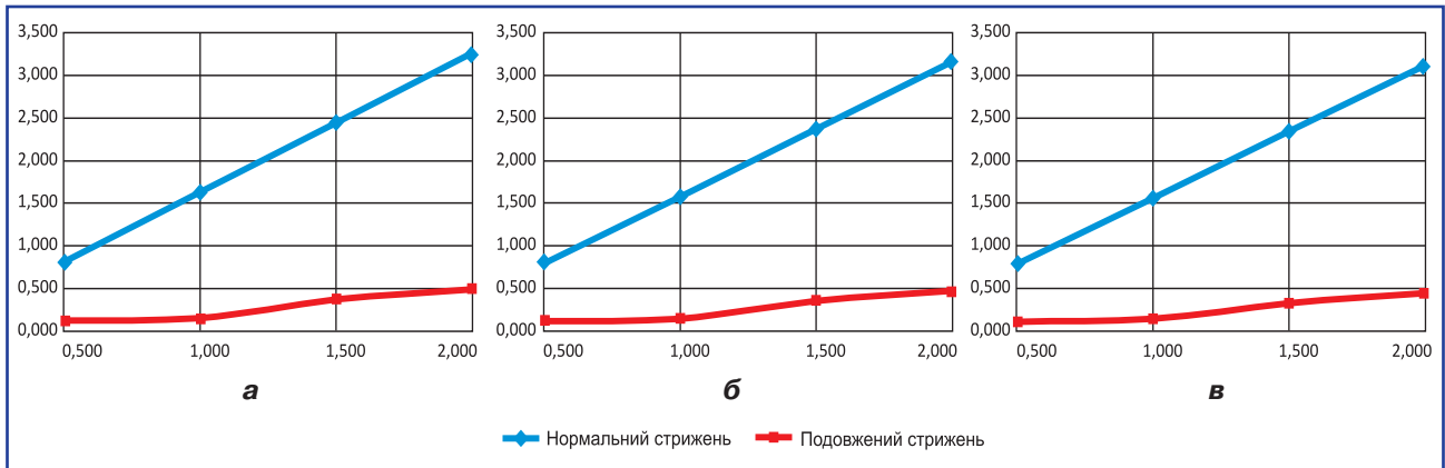
Рисунок 11. Графіки залежності показників загальних переміщень по площині перелому А3 від навантаження на кінцівку при застосуванні звичайного та подовженого проксимального стегового стрижня без блокуючих гвинтів (а), з одним блокуючим гвинтом (б) та двома блокуючими гвинтами (в)
