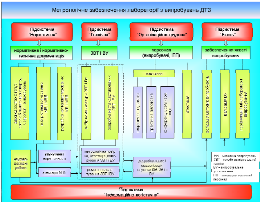
Рисунок 1 – Підсистеми системи метрологічного забезпечення лабораторії з випробувань транспортних засобів
